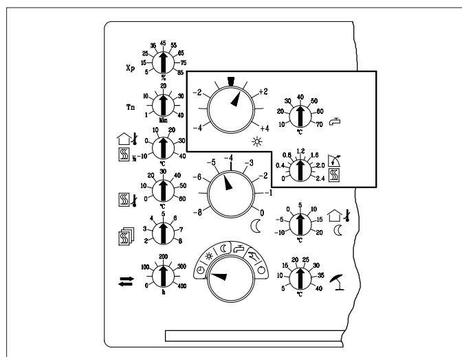
Afb. 12 Bedieningsniveau 2 van de cascaderregelaars K2R-F, K2M-F en K4BUwUw (M)
