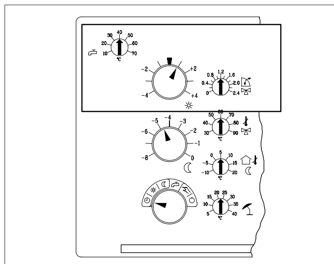
Afb. 11 Bedieningsniveau 2 van de menggroepregelaars UM en UML
