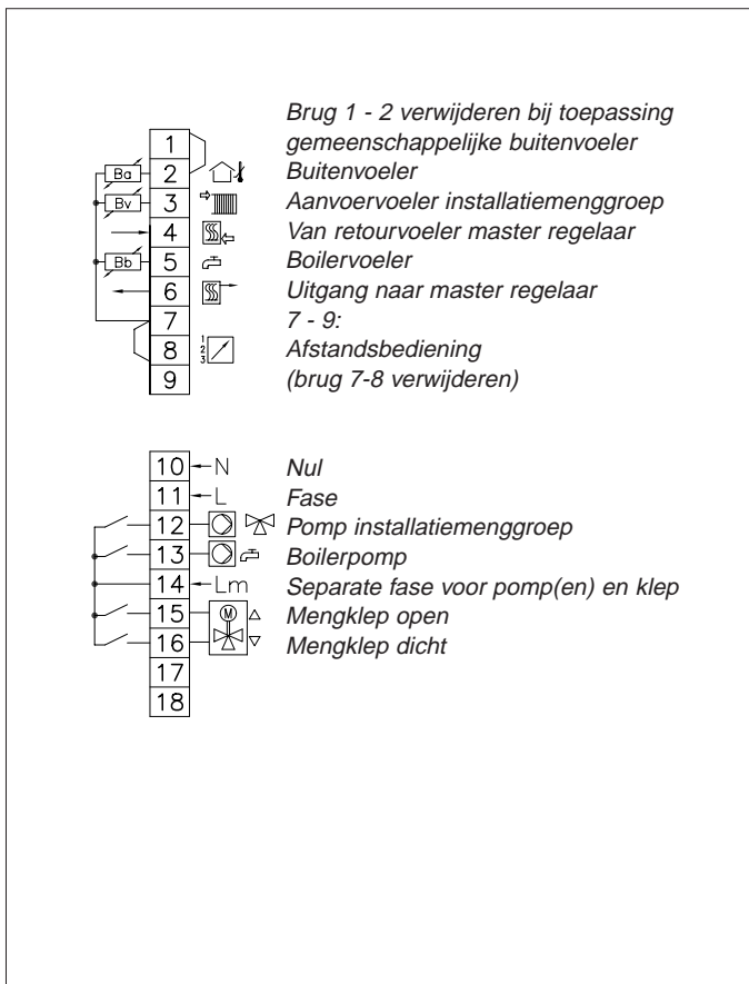
Afb. 26 2935 UML
