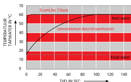
WARMWATERPRODUCTIE COMBI-KETELS
